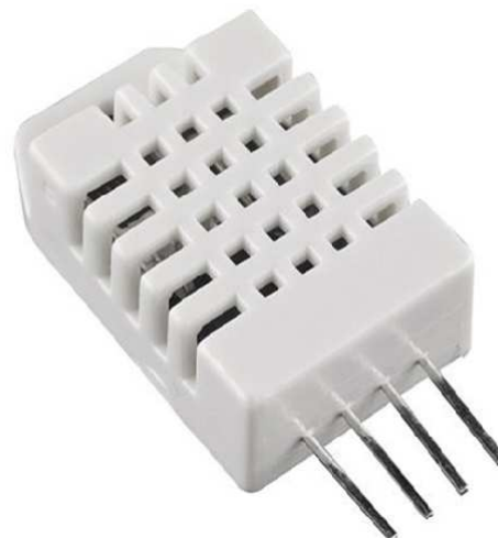
Fig.4. Sensor de humedad relativa y temperatura DHT22
